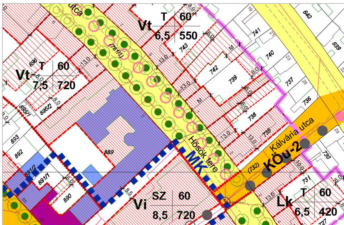
SZ-3 szabályozási terv módosított állapota
