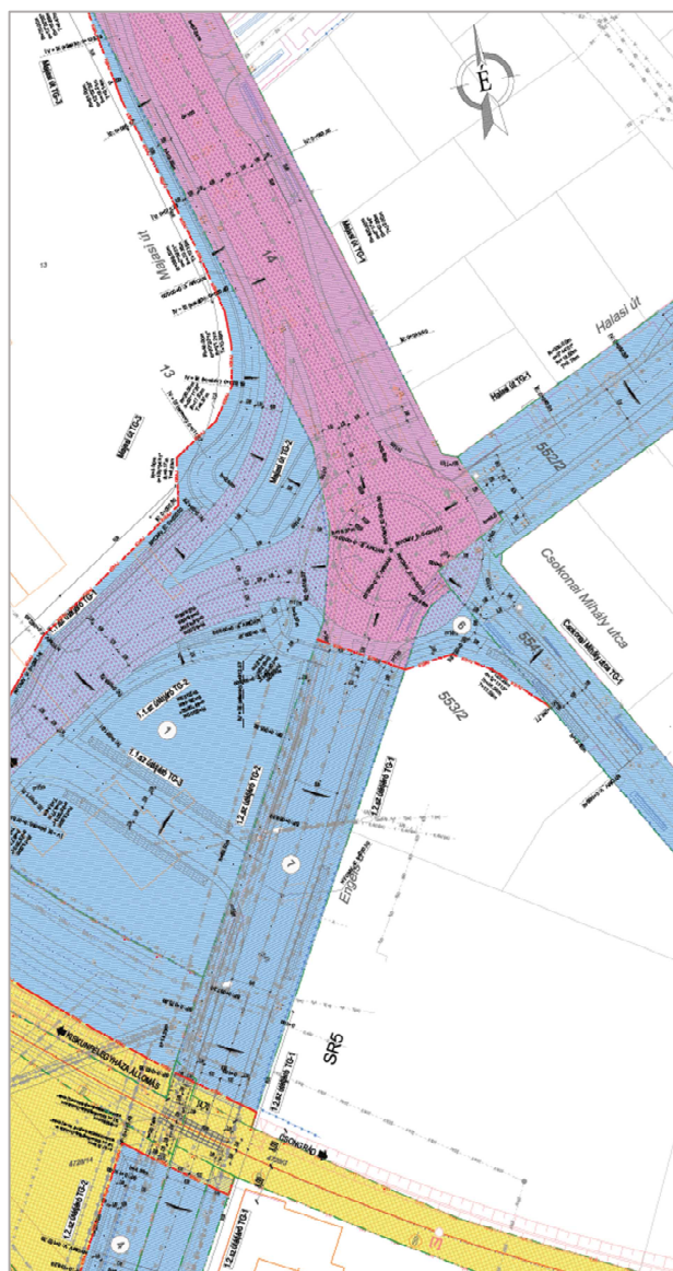
Halasi-Izsáki úti körforgalom kialakítása (Kontúr Csoport Kft. terve)
